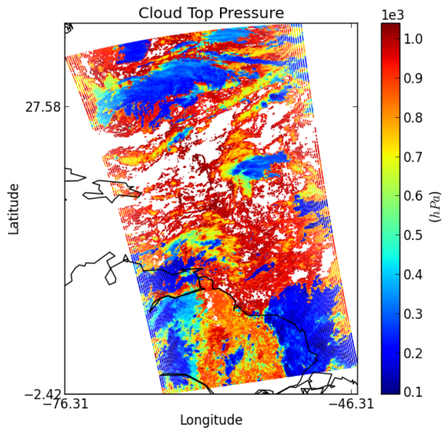
Fig. 12.3: MODIS Level 2
