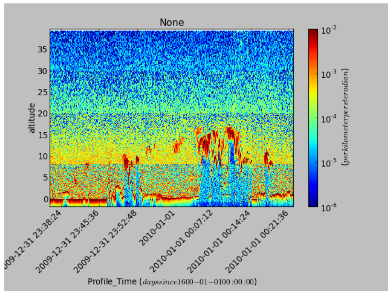
Fig. 12.12: CALIOP Level 1b
